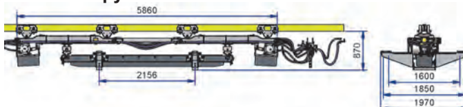
SLG 4.4 Макс. допустимая нагрузка 16.000кг*
