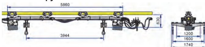
SLG 4.5 Макс. допустимая нагрузка 16.000кг*
